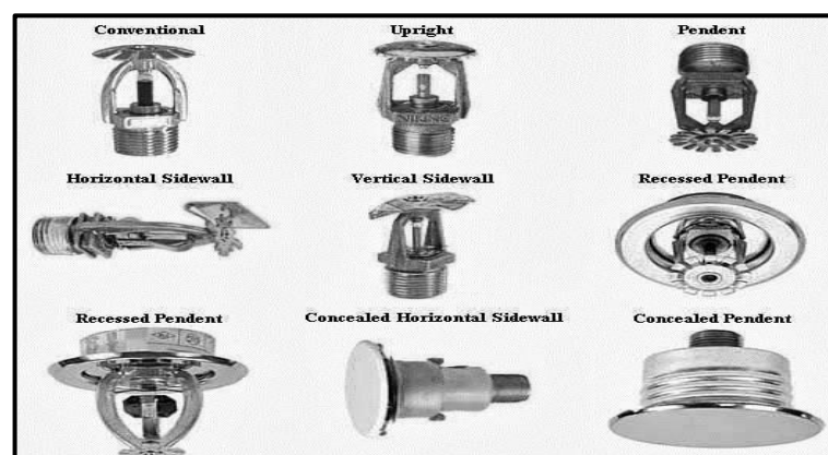
Rajah 4: Contoh Sistem Semburan Air Automatik
